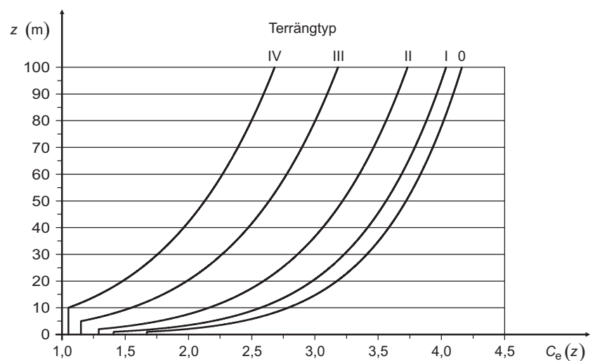
Figur C-5 Exponeringsfaktorn c_e(z) för c_0 = 1,0 och k_t = 1,0
